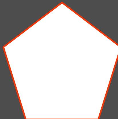
Regelmäßiges Fünfeck
