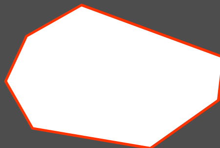
Siebeneck
