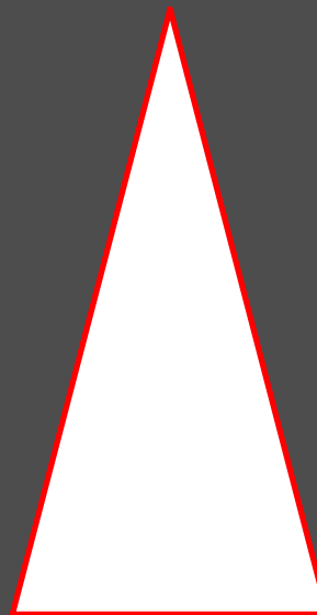
Gleichschenkliges Dreieck
