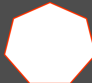
Regelmäßiges Siebeneck
