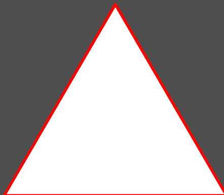
Gleichseitiges Dreieck
