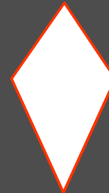
Drachenviereck
