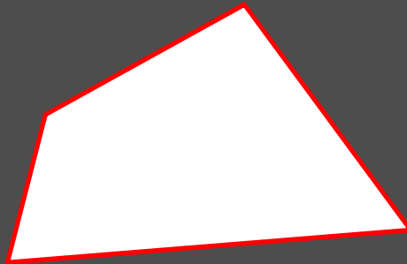
Viereck
