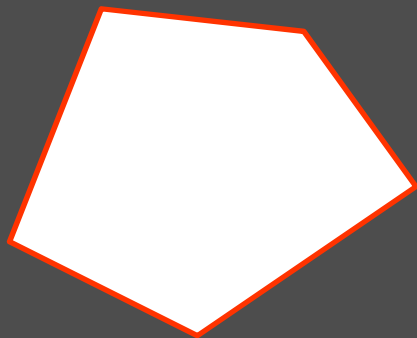
Fünfeck
