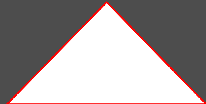
Gleichschenkliges und rechtwinkliges Dreieck
