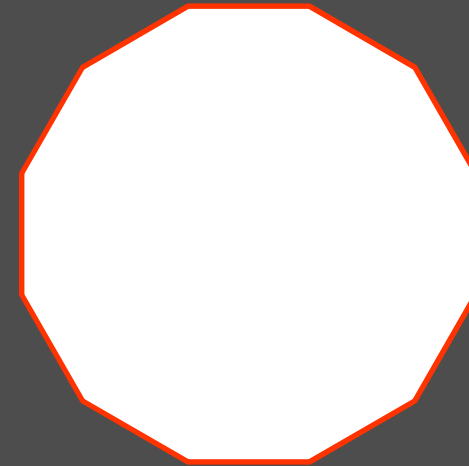
Regelmäßiges Zwölfeck
