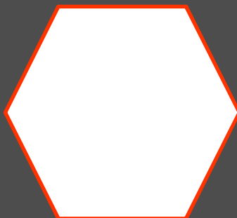
Regelmäßiges Sechseck
