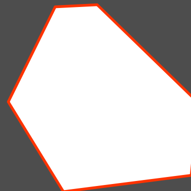
Sechseck
