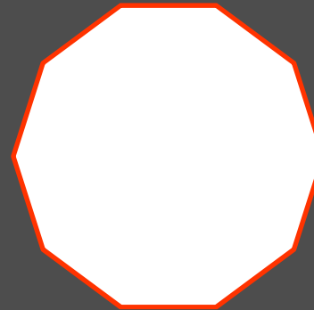
Regelmäßiges Zehneck
