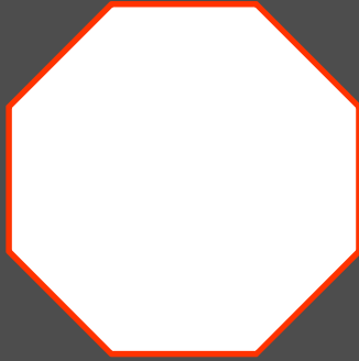
Regelmäßiges Achteck
